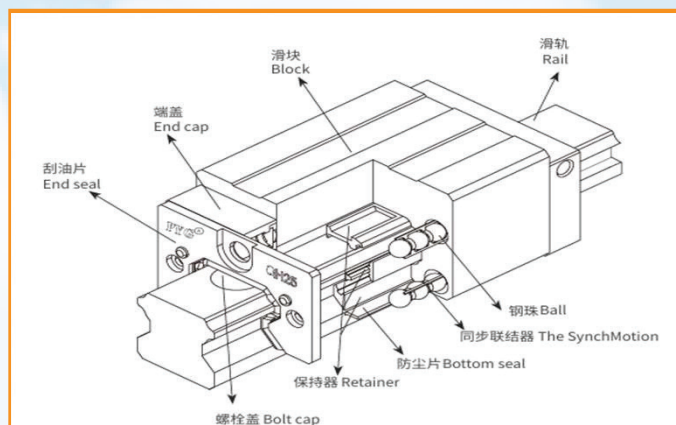
1. Con Trượt Bi Cầu, Độ Ổn Thấp, Có Vòng Cách Nhựa
