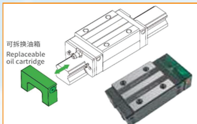
2. Con trượt tự bôi trơn, có vòng cách nhựa, độ ổn thấp
