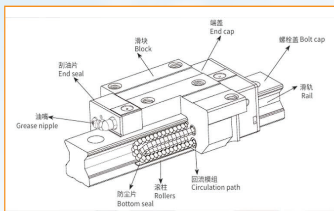
3. Con trượt bi trụ, tải nặng và độ chính xác cao
